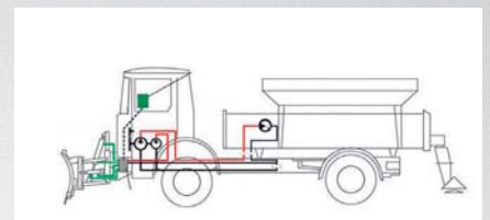
HYDRAULIKANLAGE Ein-, Zweikreis und Loadsensing Anlage
