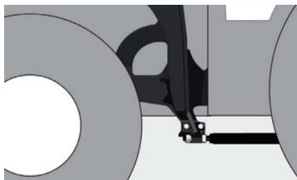
Aktive Hinterachsabstützung Vorgespannt als Unterstützung für den Traktorrahmen.
