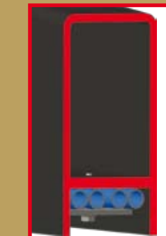
Neues Schwingenprofil, aus Feinkornstahl garantiert beste Qualität und höchste Stabilität. Verlegung der Hydraulikleitungen unterhalb der Schwinde - unsichtbar, besser geschützt, leicht zugänglich.
